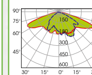
OTTICA 6 STRADALE STREET OPTIC 6
