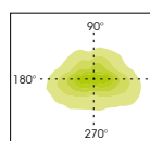
OTTICA 6 STRADALE STREET OPTIC 6
