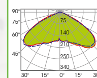
OTTICA 1 CIRCOLARE CIRCULAR OPTIC 1
