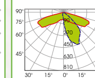
OTTICA 9 PEDONALE PEDESTRIAN OPTIC 9
