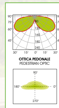
CURVA FOTOMETRICA - PHOTOMETRIC CURVE
